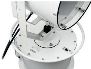
Cable Guard für Remote Unit
